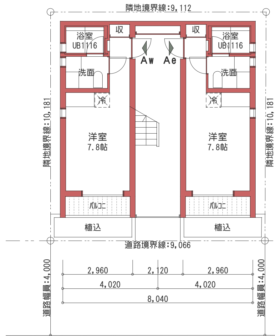
配置図・1階平面図
