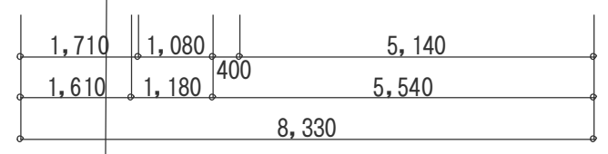
配置図・1階平面図
