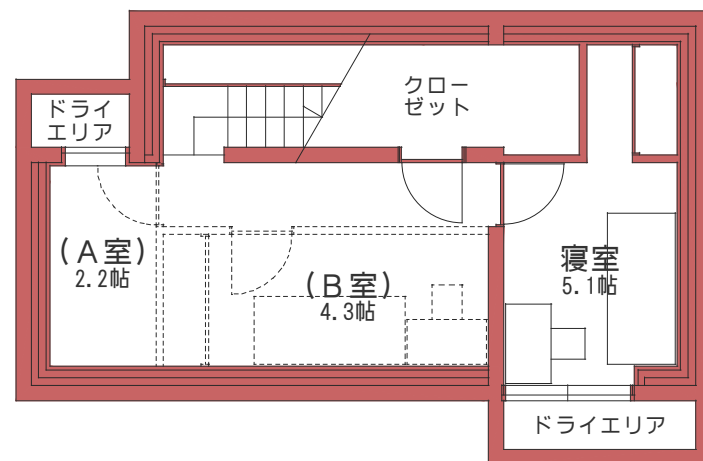
地階平面図
