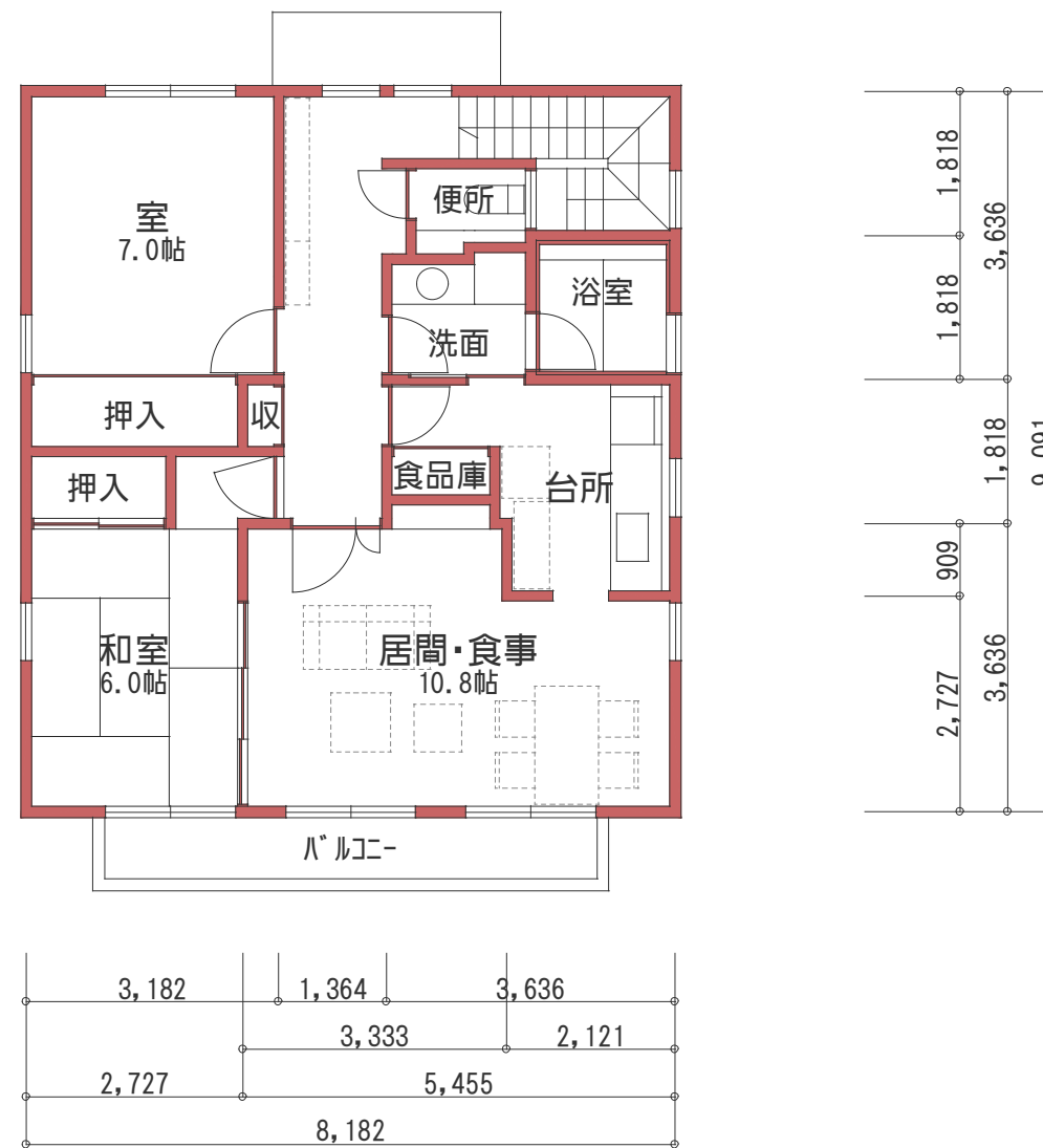
2階平面スケッチ 100 -1 床面積: 74.38㎡ [22.50坪]
